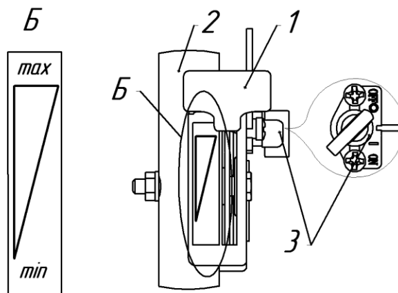
Рис.9 Дистанционное управление двигателем
